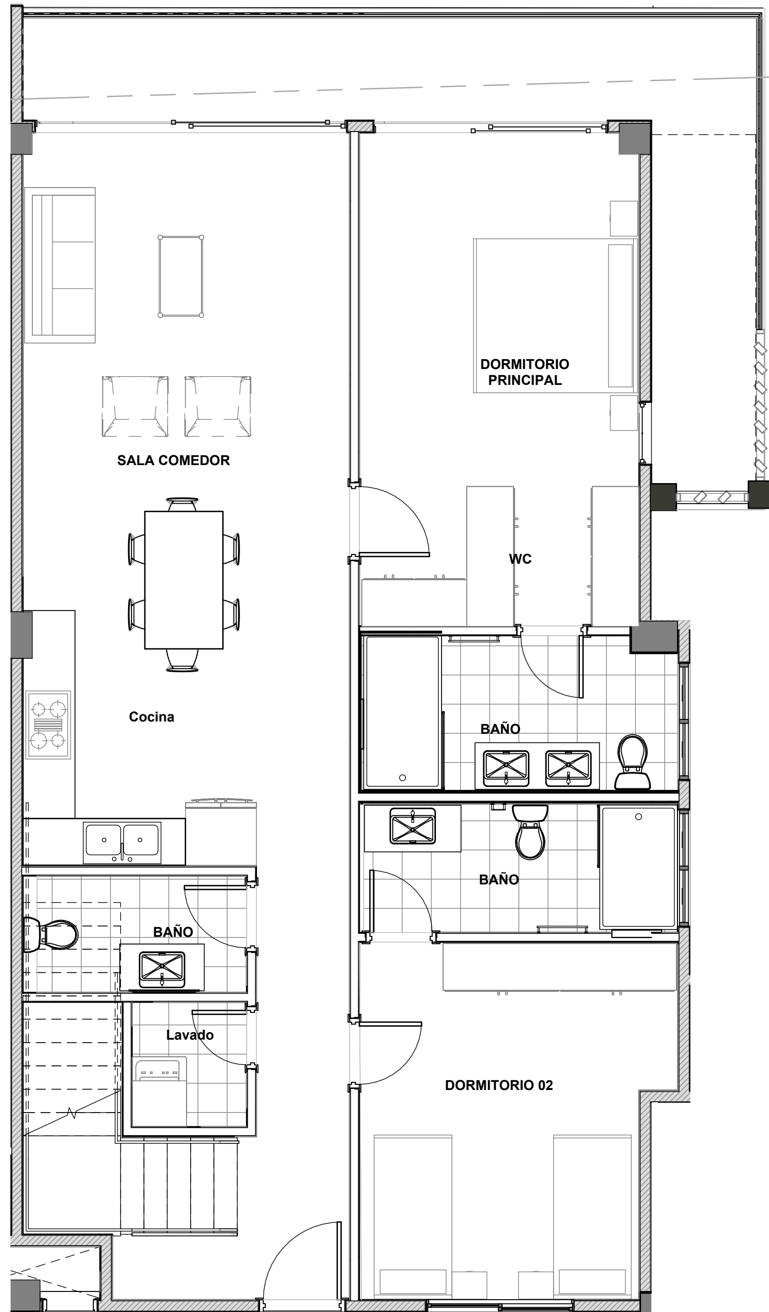
4 TIPOLOGIA F.1 (180 M2) ESC. 1 : 50
