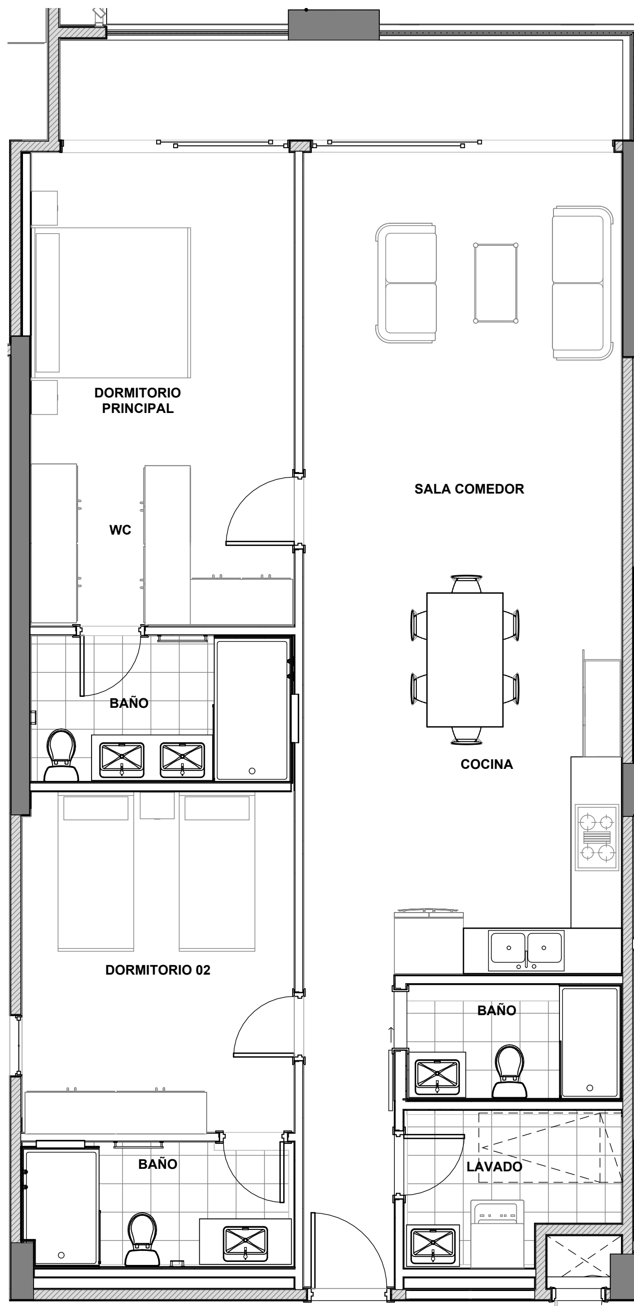
1 TIPOLOGIA D (134 M2) ESC. 1 : 50
