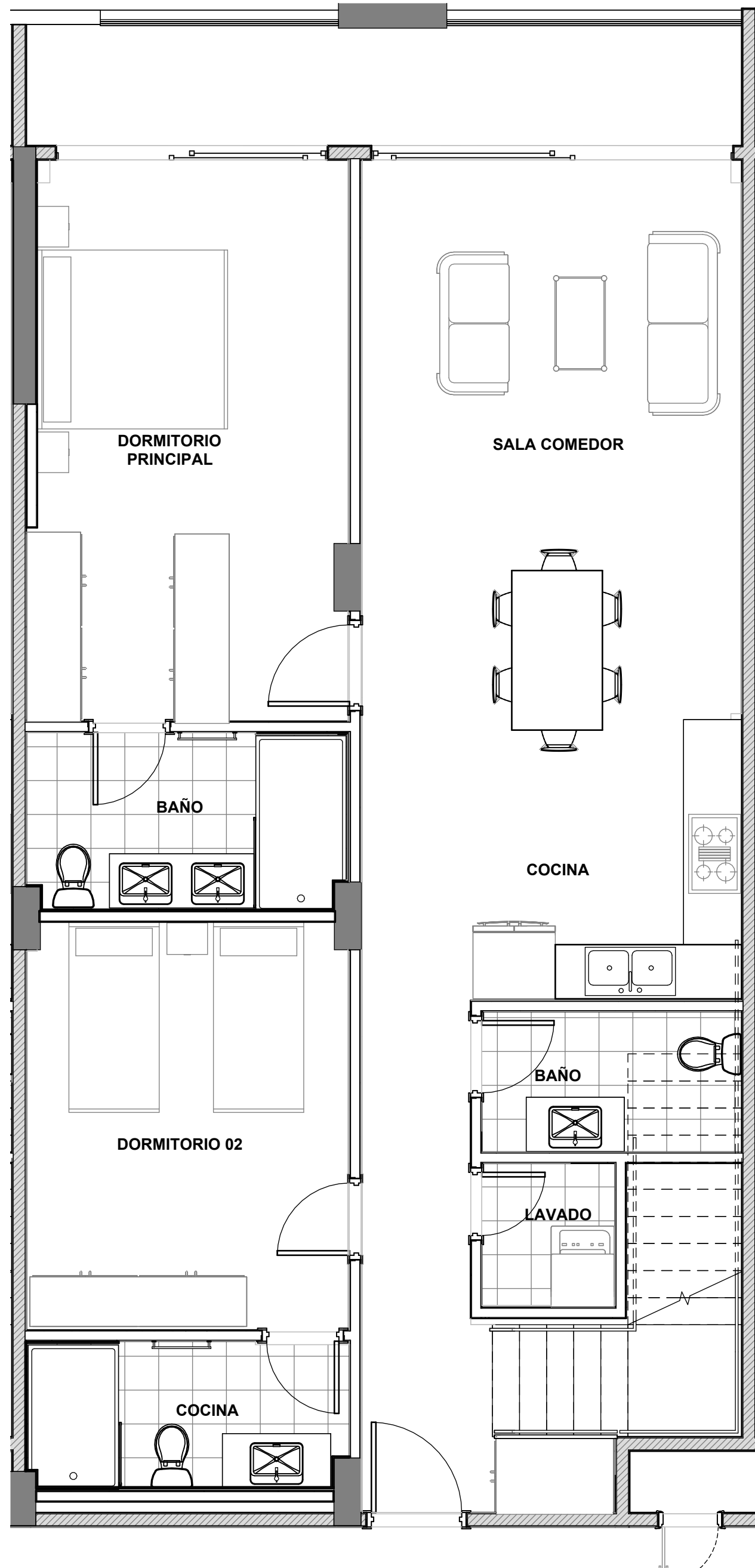
3 TIPOLOGIA F (165.48 M2) ESC. 1 : 50
